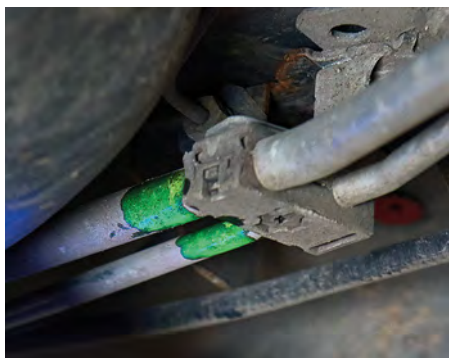
Fugas en la línea de refrigerante del aire acondicionado de vehículos mediante un agente de contraste bajo luz ultravioleta.
