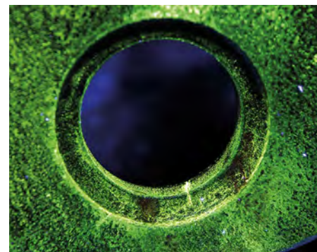
Grieta en un componente del freno de aviones mediante prueba NDT con polvo magnético bajo luz ultravioleta.
